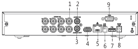
DHI-XVR5108HS-4KL
